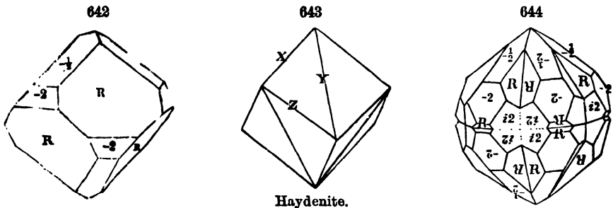
Haydenite.
